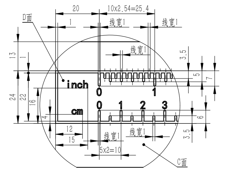
E向局部
